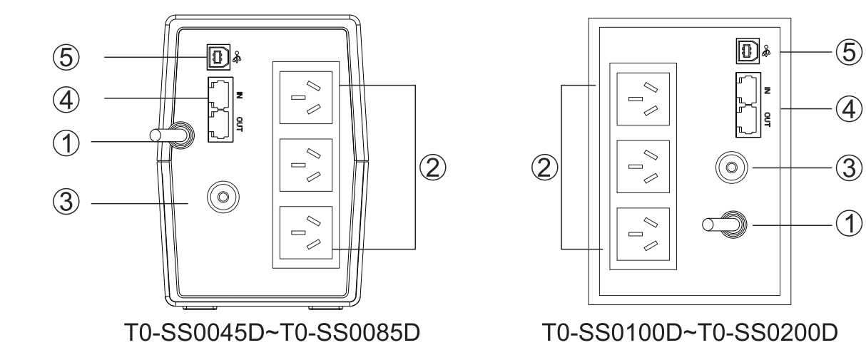
后板图
